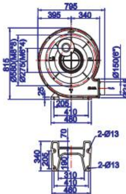
TB150L-10
