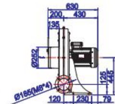
TB150-7.5 / TB150-10
